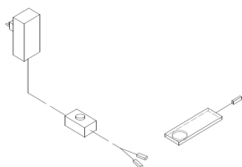
LED osvětlení 3,5 W /1 ks v sadě/ montáž na spodní stranu horní desky vitrin "teplé-bílé" světlo, včetně trafa a kabelů
