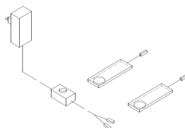
LED osvětlení 3,5 W /2 ks v sadě/ montáž na spodní stranu horní desky vitrin "teplé-bílé" světlo, včetně trafa a kabelů
